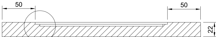
A-A (1:2)
