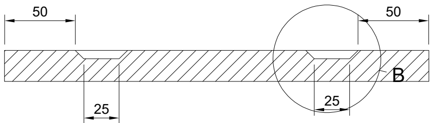
A-A (1:2)
